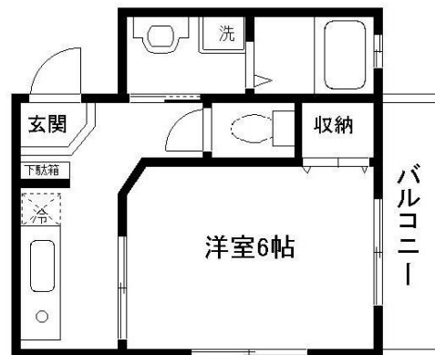
【間取り図】
